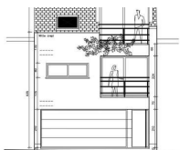
Voorgevel
